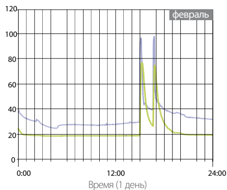
— Открытие см 2 (= Поток м 3 /ч @ 10 Па) — Относительная влажность %
