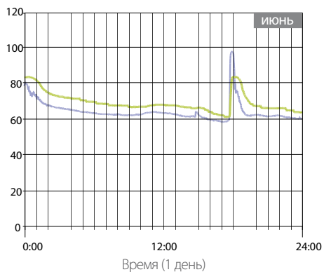
— Открытие см 2 (= Поток м 3 /ч @ 10 Па) — Относительная влажность %
