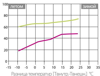
Средняя вытяжка при фиксированной решетке м 3 /ч
